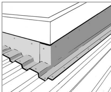
1. Scellement de la couverture avec parapets
