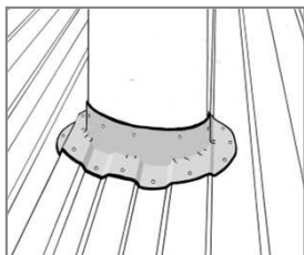
5. Selagens da cobertura com conduatas circulares
