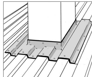
3. Selagem da cobertura com atravassamento rectangular
