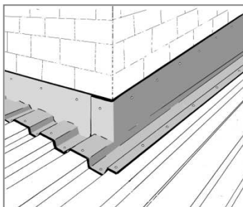
2. Selagem da cobertura com fachadas
