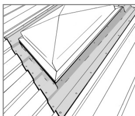
4. Selagem da cobertura com clarabóias
